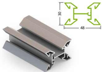
ПРОФИЛЬ НЕСУЩИЙ ВЕРТИКАЛЬНЫЙ
