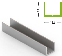
ПРОФИЛЬ П-ОБРАЗНЫЙ ГОРИЗОНТАЛЬНЫЙ
